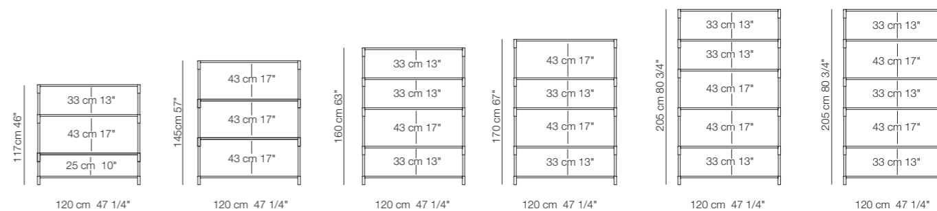
Composizioni librerie Bookcases compositions
